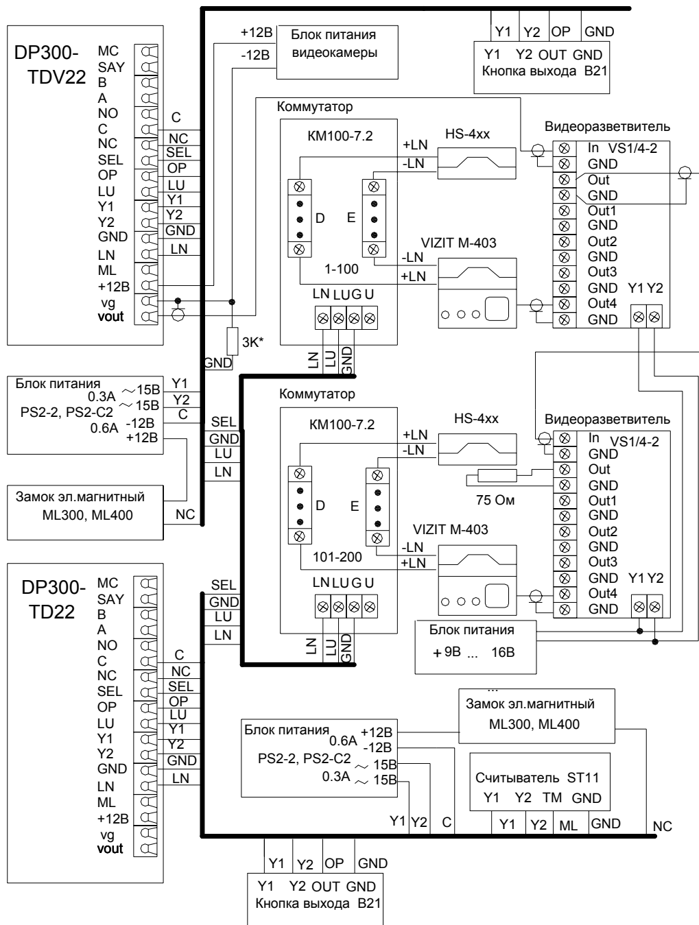
Рис.3 Пример схемы подключения DP300-TDV22 в составе домофонного комплекса.
