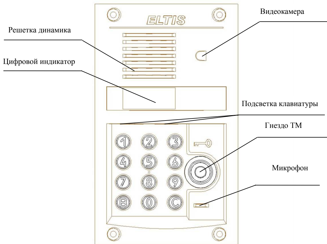
Рис.1 Внешний вид со стороны лицевой панели блока вызова DP300-TDV22.
